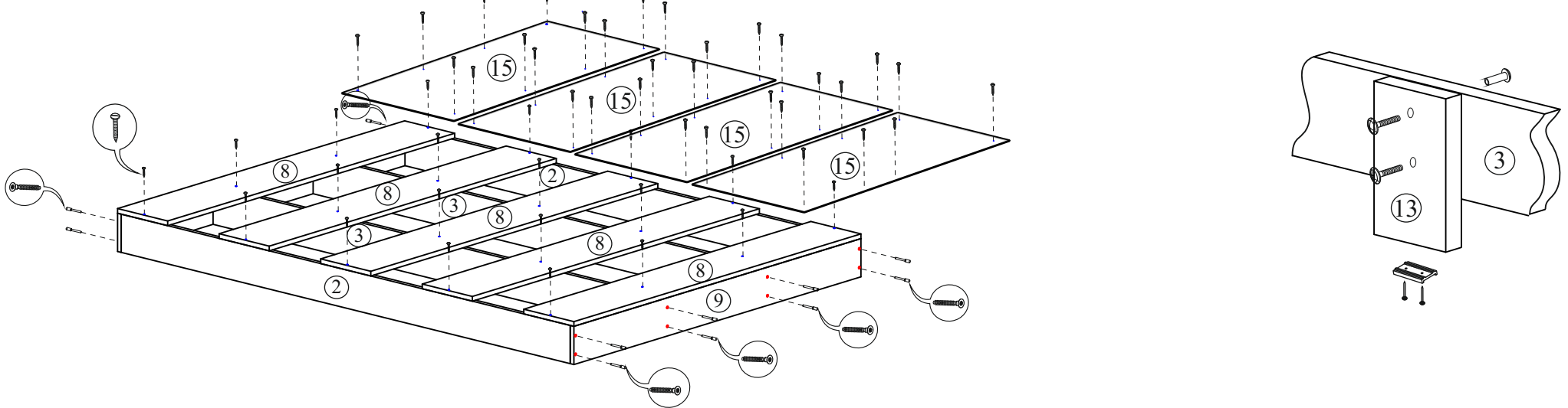
Монтаж эксцентриковой стяжки
